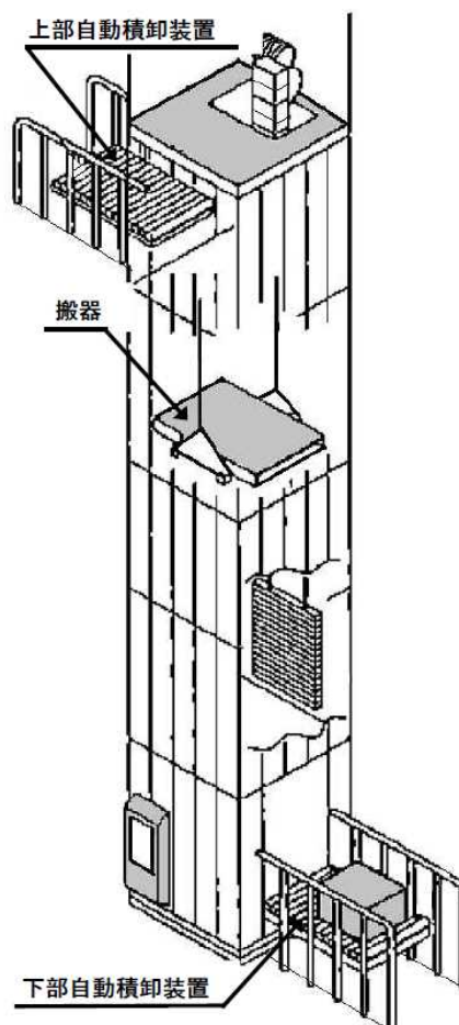
図 1 垂直自動搬送機の例
